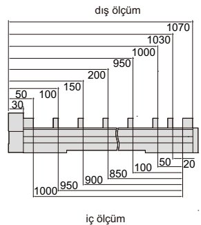
dış ölçüm
