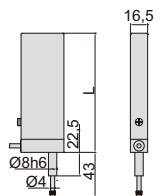
Ünite: mm
