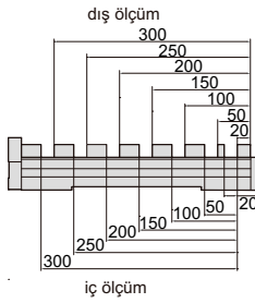
dış ölçüm
