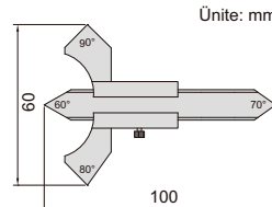
Ünite: mm
