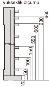
yükseklik ölçümü
