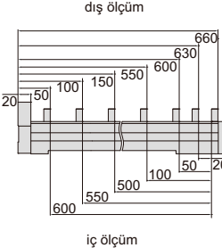
dış ölçüm
