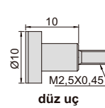
düz uç
