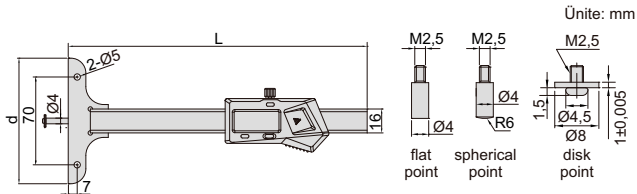
küçük deliklerin (>Ø4mm) derinlik ölçümü
